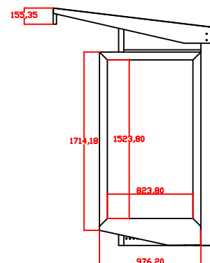
VISTA DIREITA
