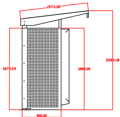
VISTA ESQUERDA
