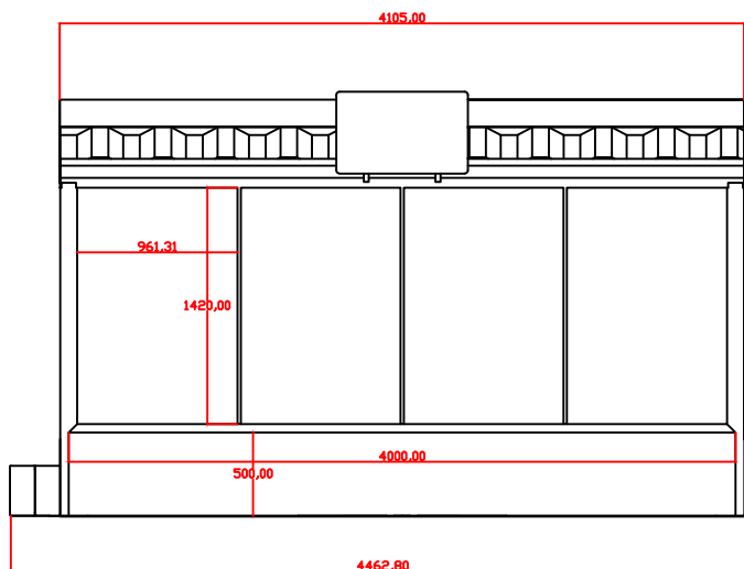
VISTA POSTERIOR
