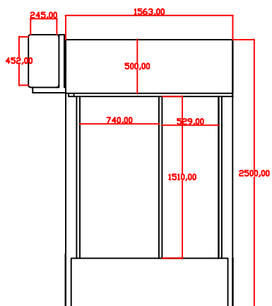
VISTA DIREITA
